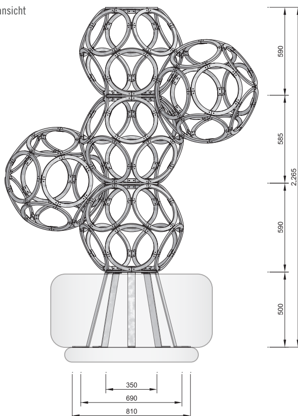
Seitenansicht
