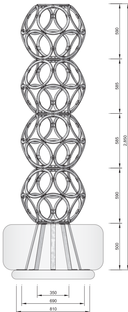
Seitenansicht
